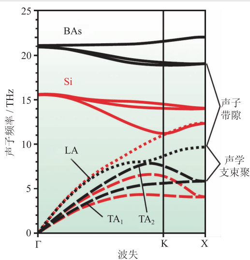
图1 硅与砷化镓的声子谱。与硅相比,砷化镓具有的声子带隙与声学支束聚增加了声子平均自由程,从而提高了热导率
